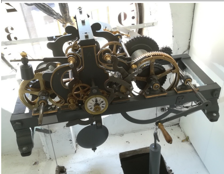
Mecanisme restaurat amb la nova pesa de la soneria. (05-07-2020)
